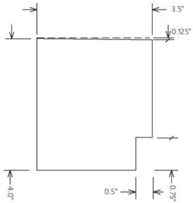
60" HBSC60 / 84" HBSC84
